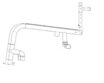
Telaio Standard vs. Telaio Lungo La differenza è 20 mm
